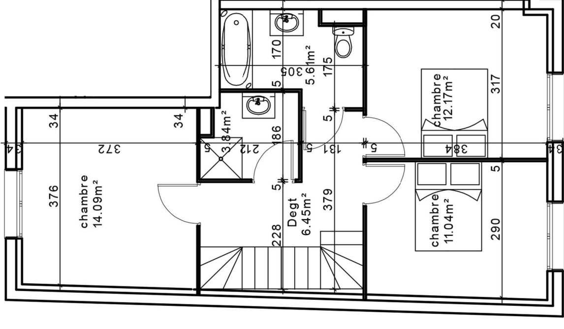
1er Etage
